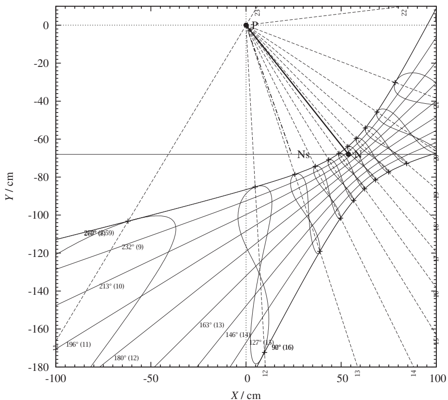
* vektorový výstup z výpočtu "SHC — návrh číselníku slunečních hodin" http://mail.astrophk.cz/~mira/shc/shc.php?lang=cz
