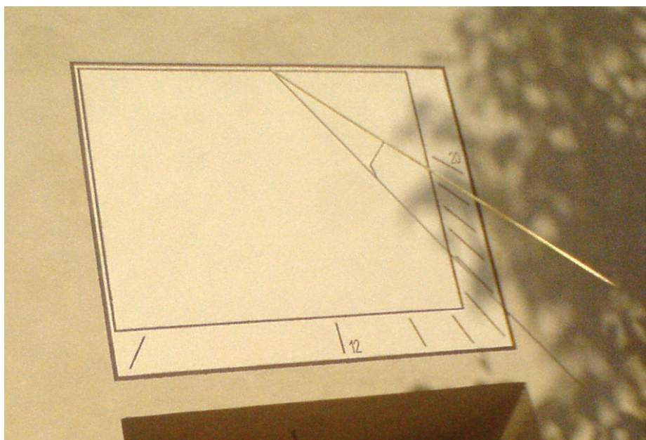
× JZ vertikální hodiny, šikmý polos, polos rovnoběžný se zemskou osou, zde úhel 49^\circ , polos směřuje k jihu, zde odklon od jihu 66^\circ , hodinové rysky od 11 do 20 hodin, ukazují středoevropský zimní čas, foceno v 16.58
